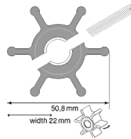
JOHNSON F4 IMPELLER (MC97) A09-810B-1 25.33 A18653-0001 21.91 JABSCO
