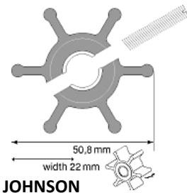
JOHNSON F4 IMPELLER ( MC97) A09-810B-1 23.02 A18653-0001 21.91 JABSCO
