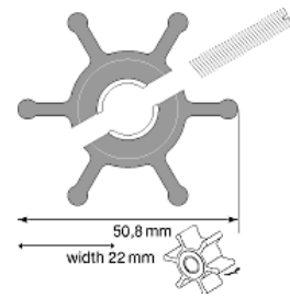
F4 IMPELLER ( MC97) JOHNSON (09-810B-1) 21.78 JABSCO 18653-0001 29.51
